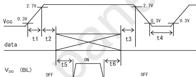
【Note6-1】 入力電圧シーケンス V CC turn-on/off conditions
